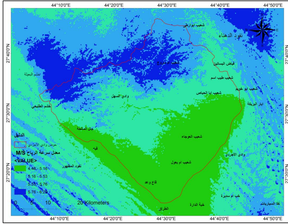
الشكل 3: سرعة الرياح السائدة في منطقة الدراسة على ارتفاع 100 متر من عام 2009 حتى 2016
